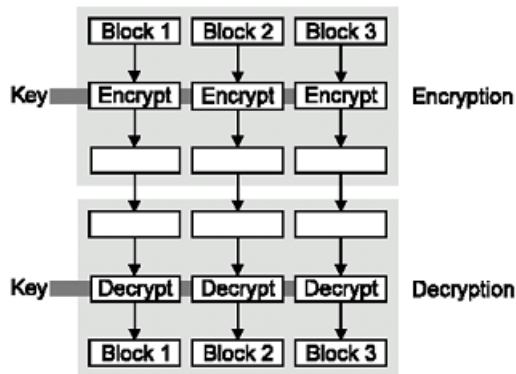
Mode ECB
